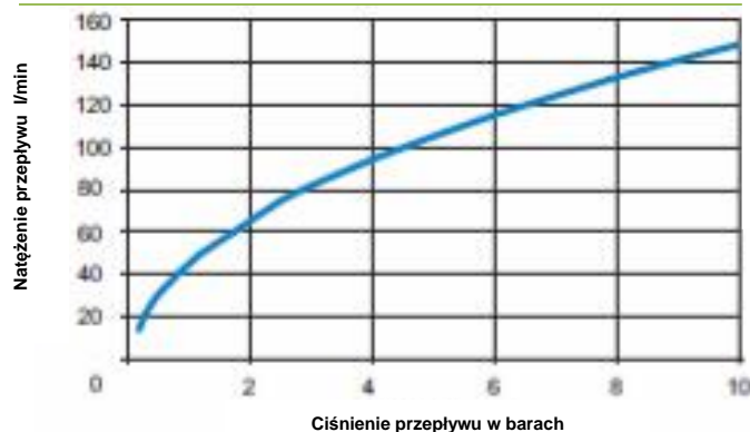
Wykres przepływu
